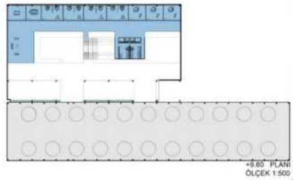
+6.80 PLANI ÖLÇEK 1:500
