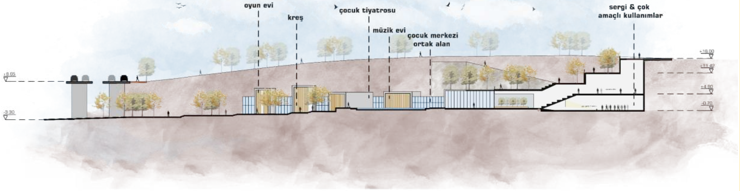
A-A Kesiti
