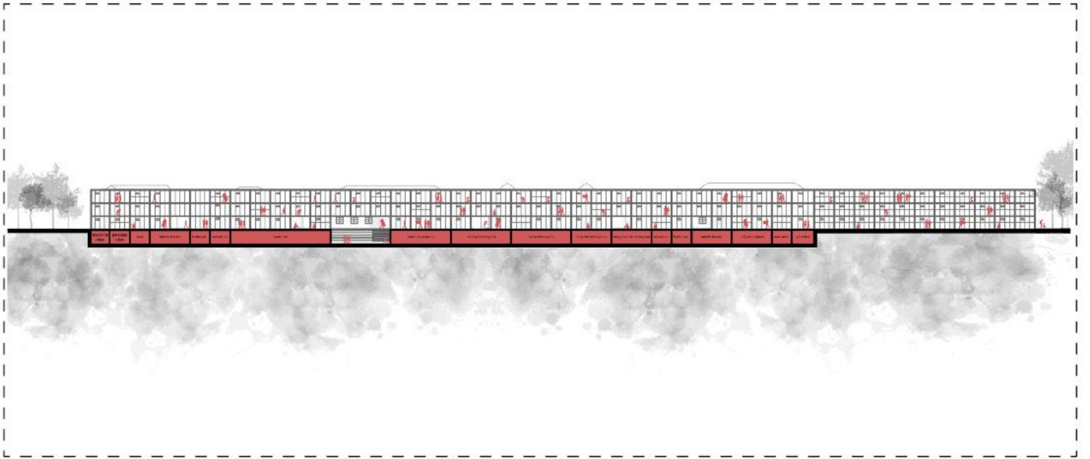
G-G Kesiti
